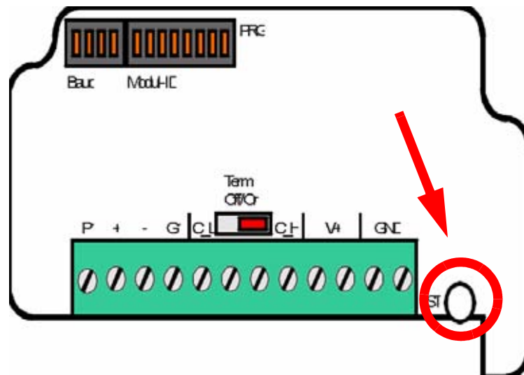
Abb. 13: Lage der LED auf dem Modul
