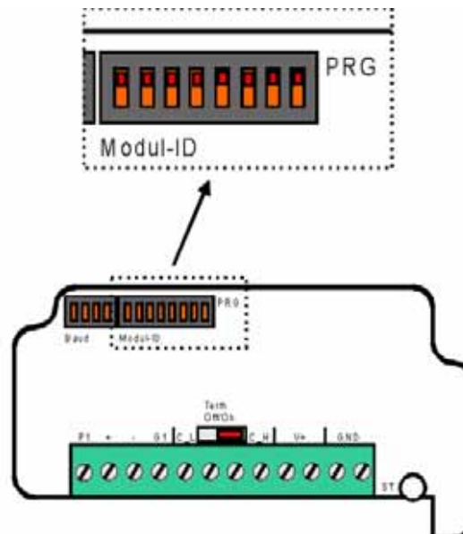
Abb. 8: DIP-Schalter, Moduladresse
