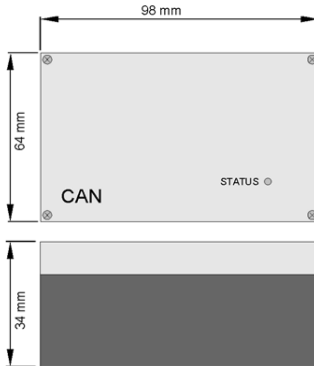
Abb. 3: Bemaßung \mu CAN.1.ti/ai
