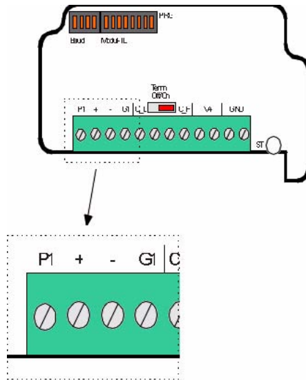
Abb. 11: Ansicht des Analogeingang
