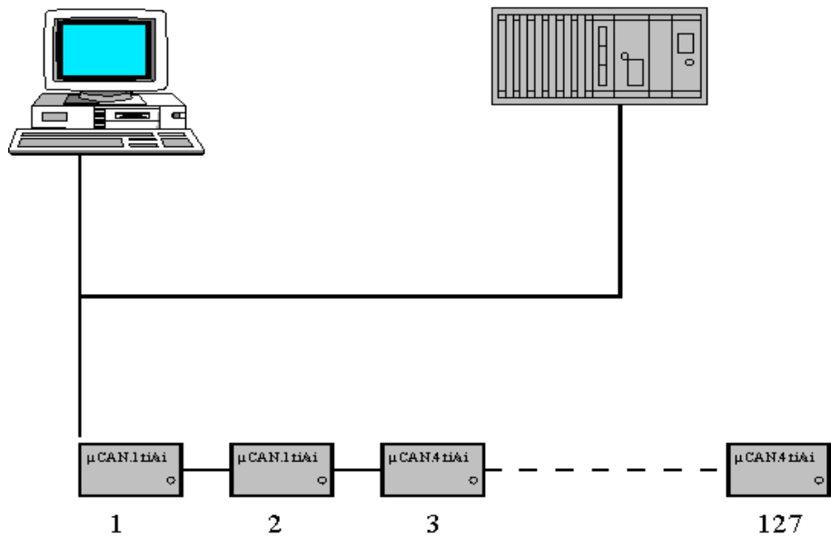
Abb. 2: Maximaler Systemausbau
